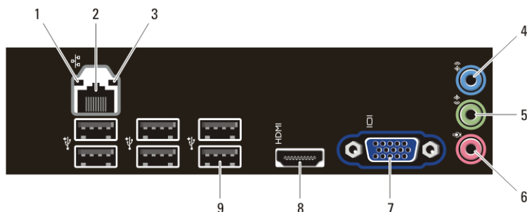
図 3. ミニタワーおよびスリムタワーの背面パネル図
