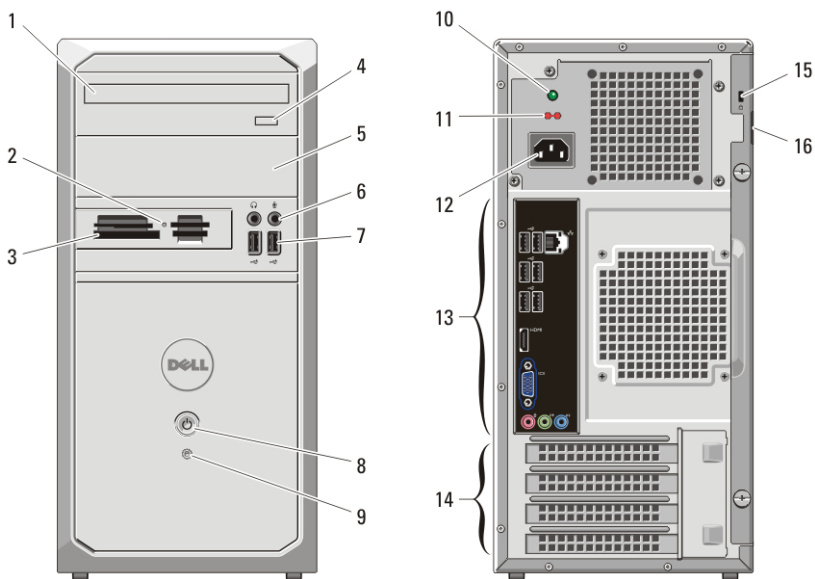
図 1. ミニタワーの正面図と背面図
